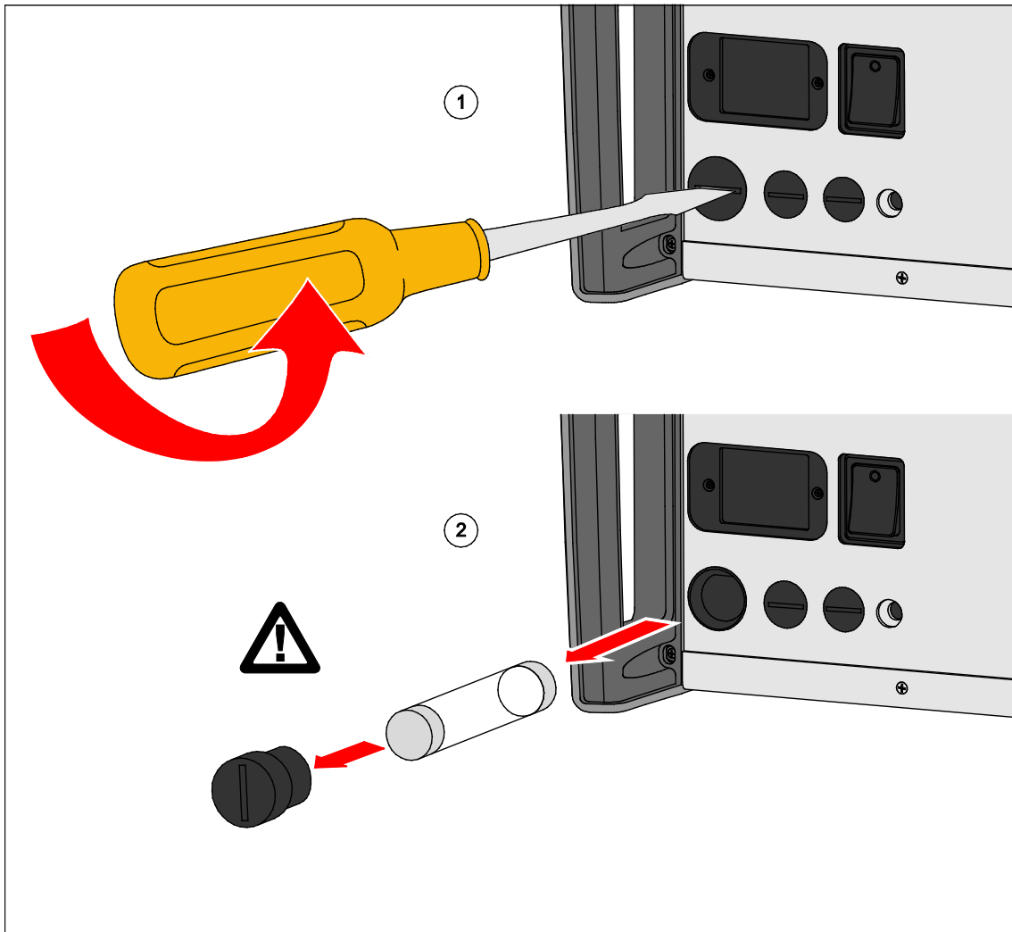
图 5-4. 更换保险丝
