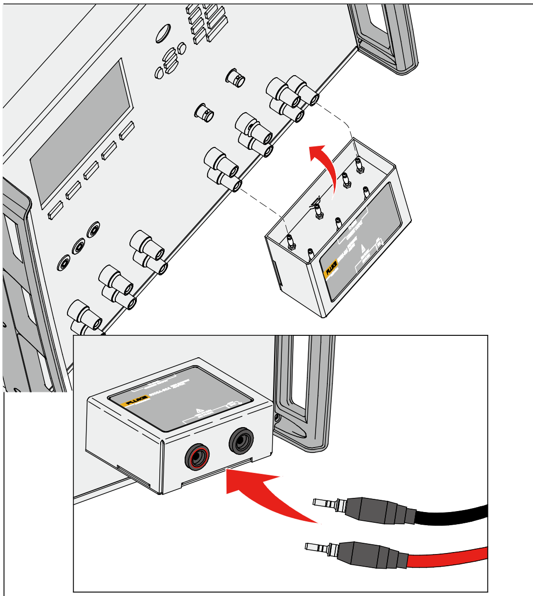
图 2-1. 配有 组合大电流适配器的产品
