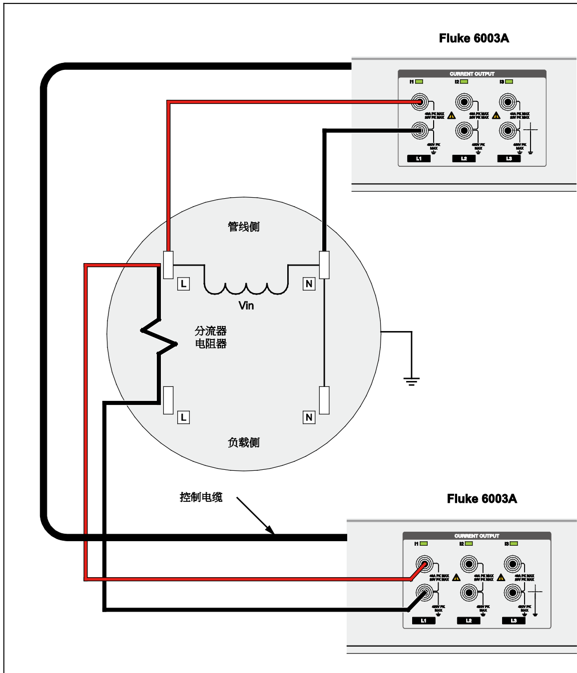
图 4-1. 隔离浮动电流输出
